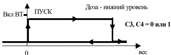
Рис. 16.2. Временная диаграмма для ВТ3 и ВТ4.
