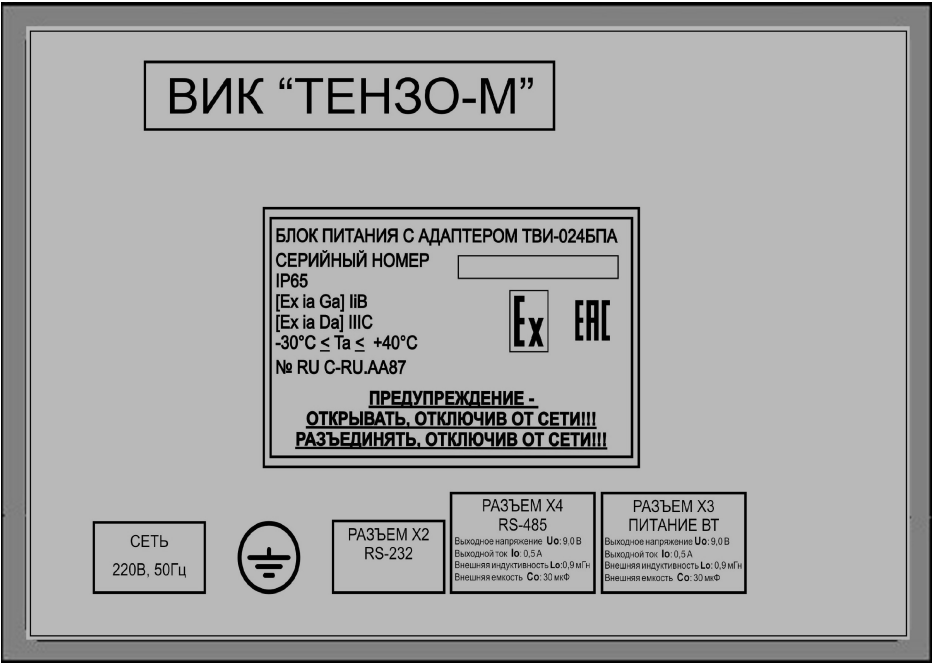
Рис. 8.4. Лицевая панель блока питания БПА.
