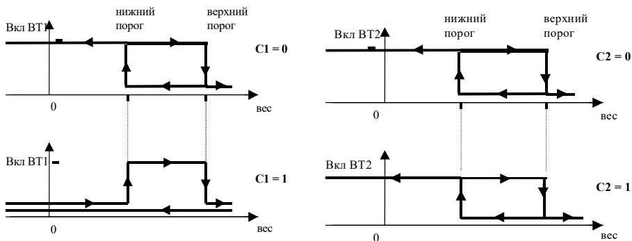
Рис. 16.1. Временная диаграмма для ВТ1 и ВТ2.
